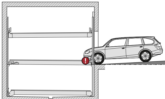
Pendiente máx. de descenso 3%
